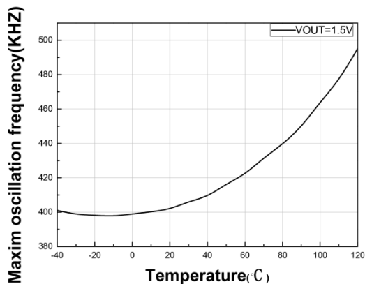
9. 振荡频率 VS 温度
