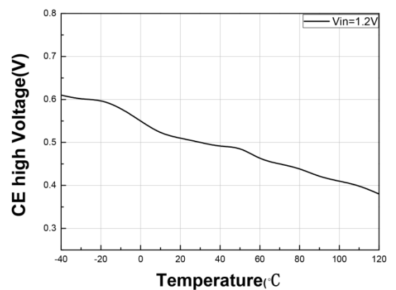
12. CE 端开启电压 VS 温度
