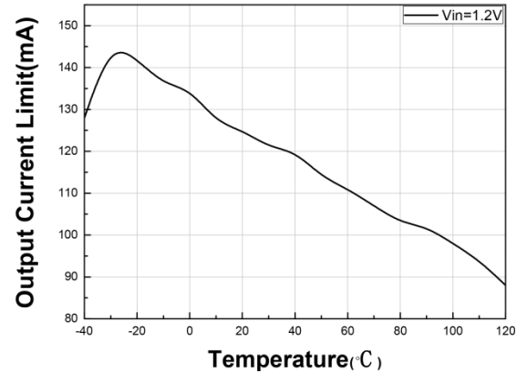
8. 带载能力 VS 温度
