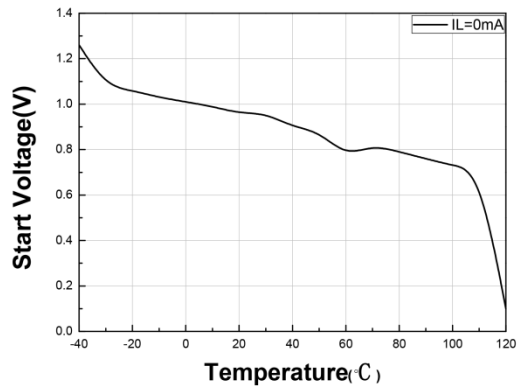
7. 启动电压 VS 温度
